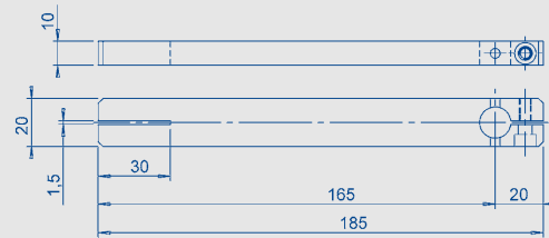
配套安装法兰托盘Z-IPX-M31
